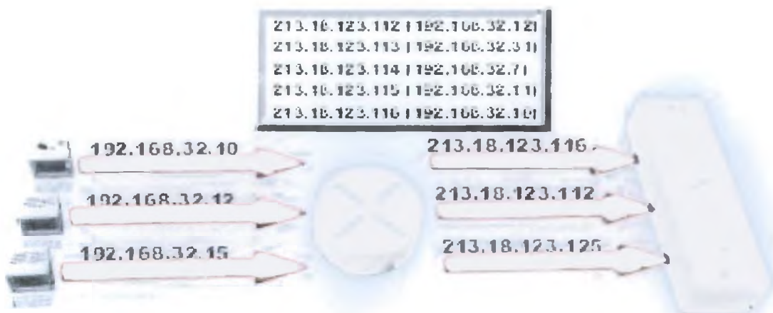
Σχήμα 12. Στην Dynamic NAT, η διεύθυνση του υπολογιστή 192.168.32.10 θα μεταφράζεται στην πρώτη διαθέσιμη διεύθυνση από 213.18.123.100 έως 213.18.123.150.
