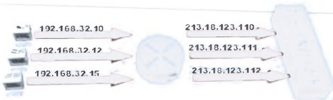
Σχήμα 11. Στην στατική NAT, η διεύθυνση του υπολογιστή 192.168.32.10 θα μεταφράζεται πάντα ως 213.18.123.110.
