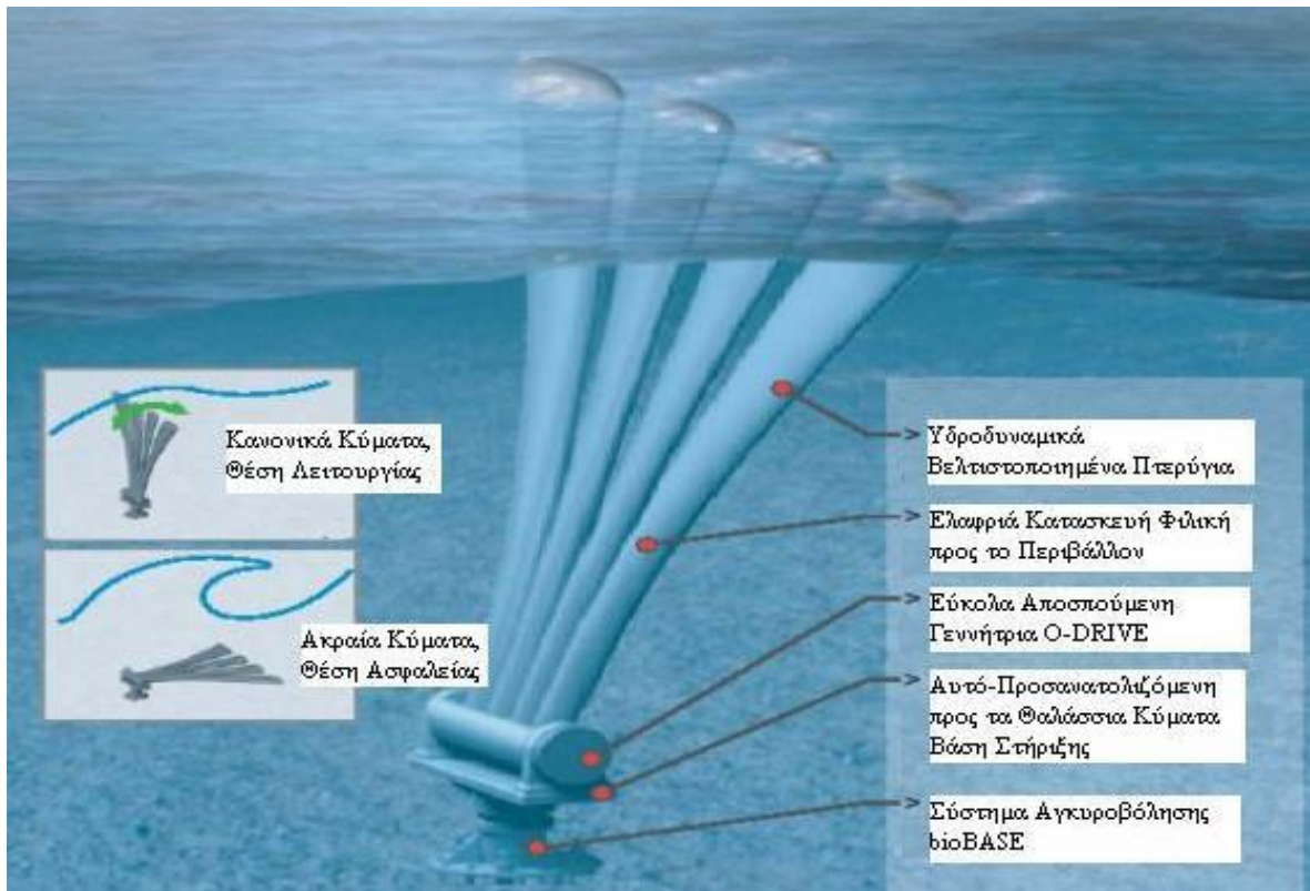
Εικόνα 4.40: Τα βασικά τμήματα του bioWAVE και οι θέσεις λειτουργίας και ασφαλείας.
