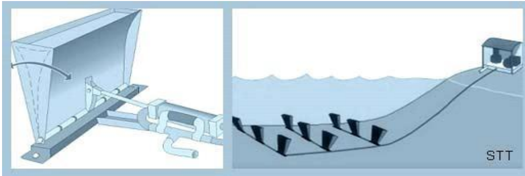
Εικόνα 4.35: Απεικόνιση τεχνολογίας οριζόντιας κίνησης με υδραυλικές αντλίες.
