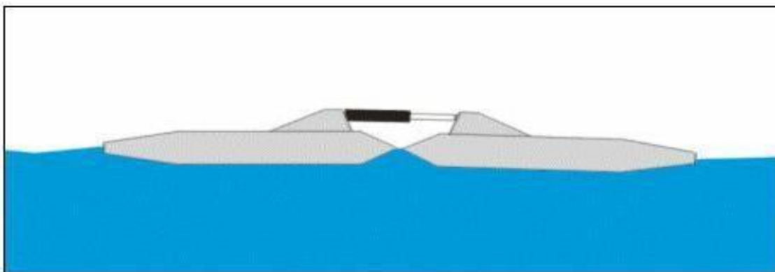
Εικόνα 4.31: Το πρωτότυπο σύστημα Cockerell Raft του 1980.
