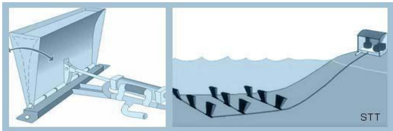
Εικόνα 4.39: Τα βασικά τμήματα ενός μετατροπέα και μιας τοπικής εγκατάστασης παραγωγής ηλεκτρικής ενέργειας με υποενοτήτες μετατροπέων.
