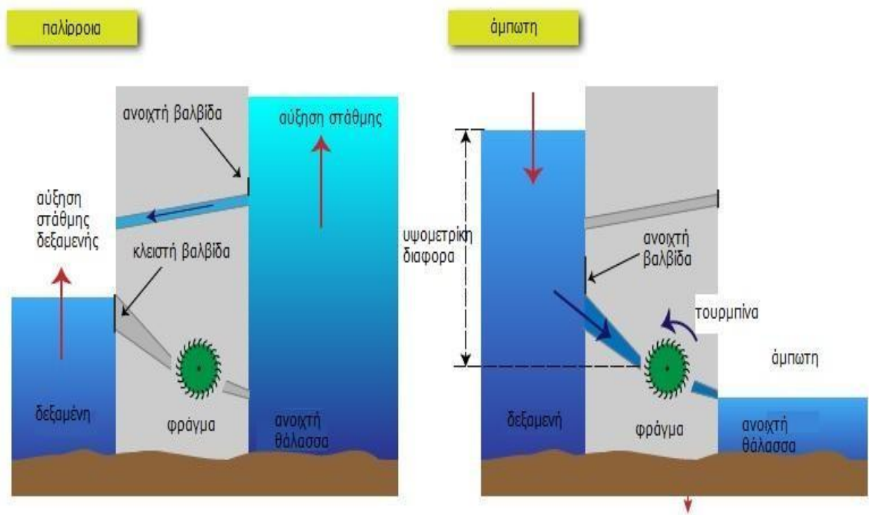
Εικόνα 2.1: Εκμετάλλευση παλίρροιας με φράγμα.
