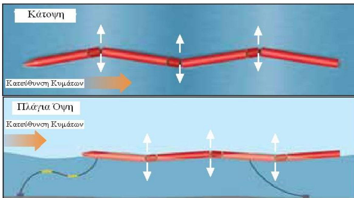
Εικόνα 4.28: Η κίνηση του μετατροπέα Pelamis τόσο ως προς τον οριζόντιο όσο και ως προς τον κατακόρυφο άξονα.
