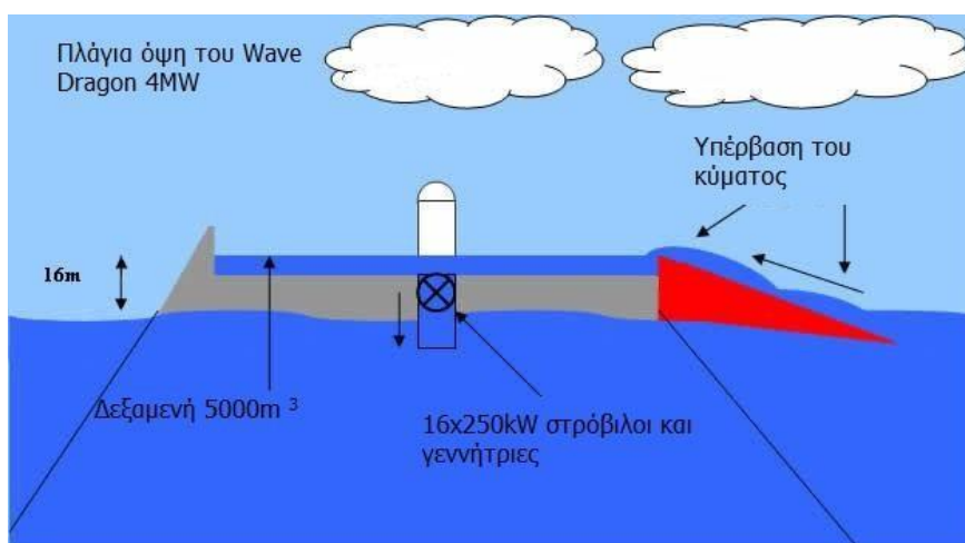
Εικόνα 4.12: Πλάγια όψη του Wave Dragon 4 MW.
