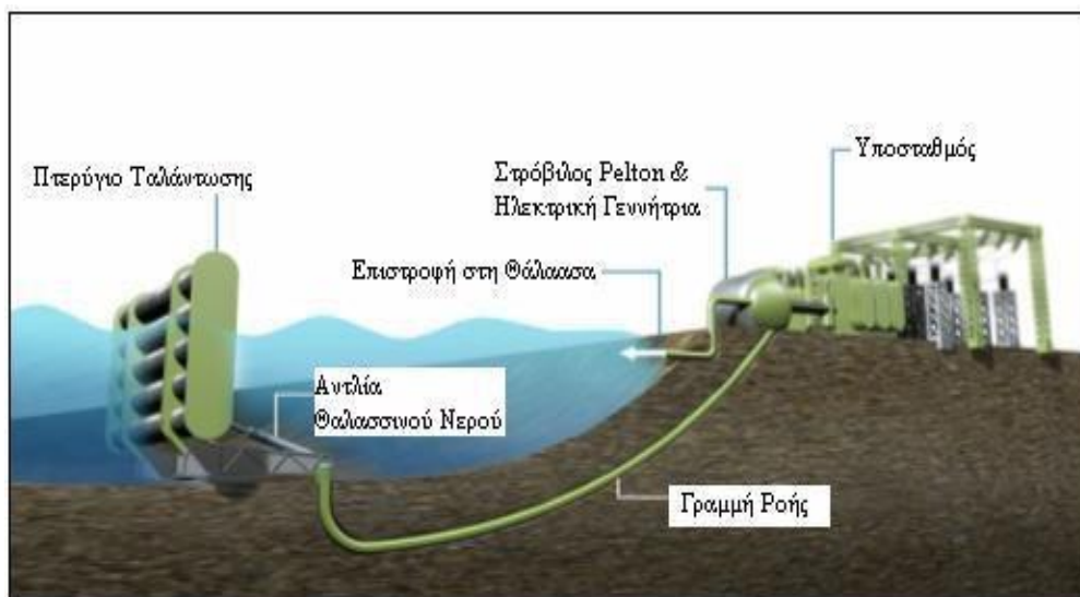
Εικόνα 4.37: Σχηματικό διάγραμμα του συστήματος μετατροπής της κυματικής ενέργειας Oyster.
