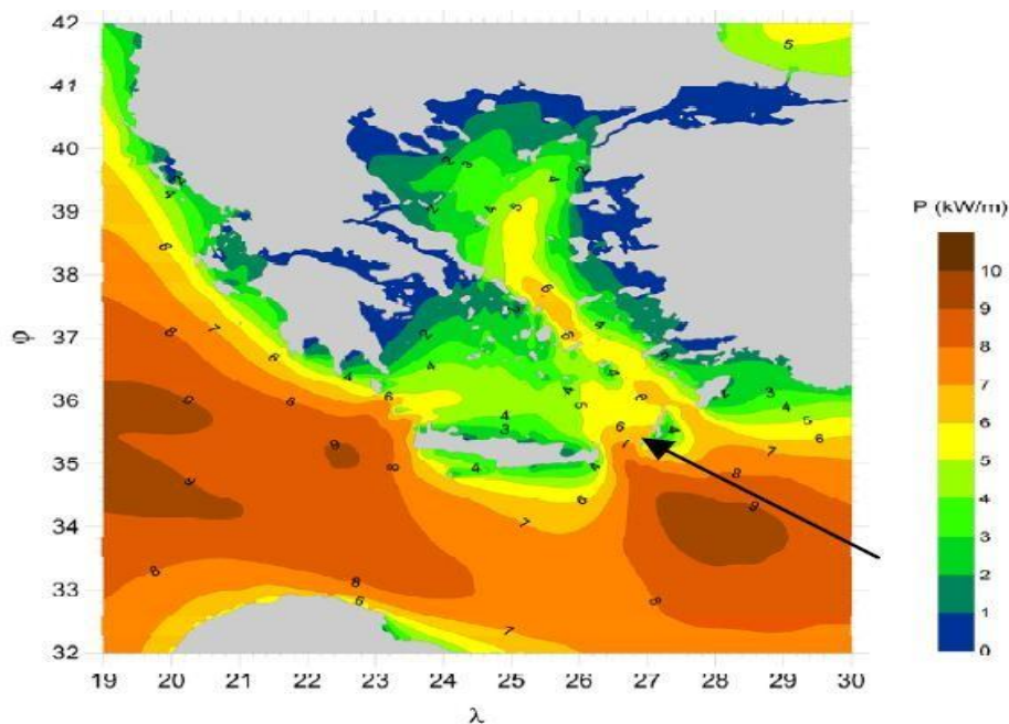
Εικόνα 5.2: Μέση κυματική ενέργεια σε ετήσια βάση των ελληνικών θαλασσών.
