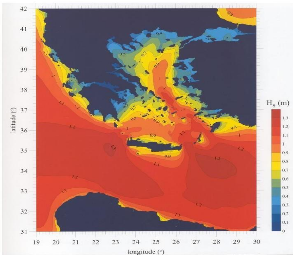
Εικόνα 5.5: Χωρική κατανομή του μέσου κυματικού ύψους H_s σε m.
