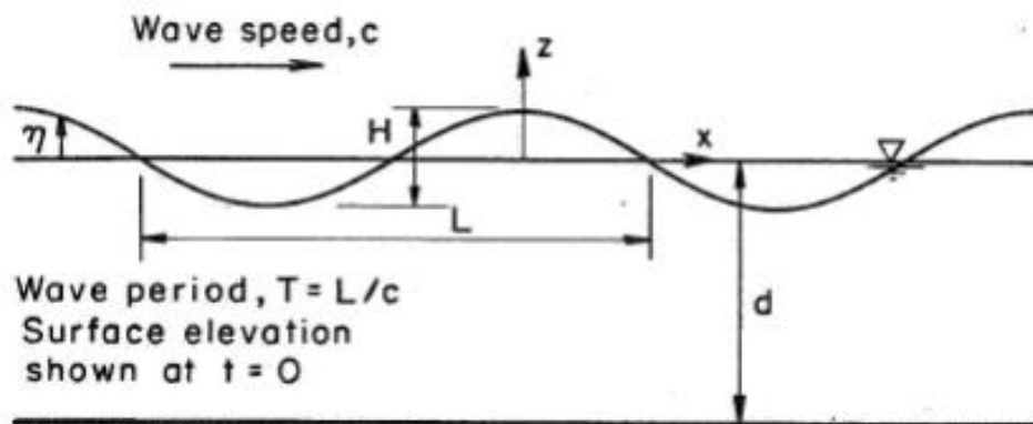
Εικόνα 1.2: Χαρακτηριστικά θαλάσσιου κύματος.
