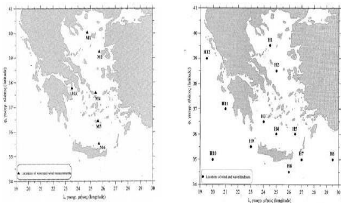
Εικόνα 5.4: Σημεία στις ελληνικές θάλασσες για τα οποία υπάρχουν κυματικά δεδομένα. Τα σημεία (M) είναι σηματοδότες παρατήρησης ενώ τα σημεία (H) είναι δεδομένα αριθμητικής προσομοίωσης.
