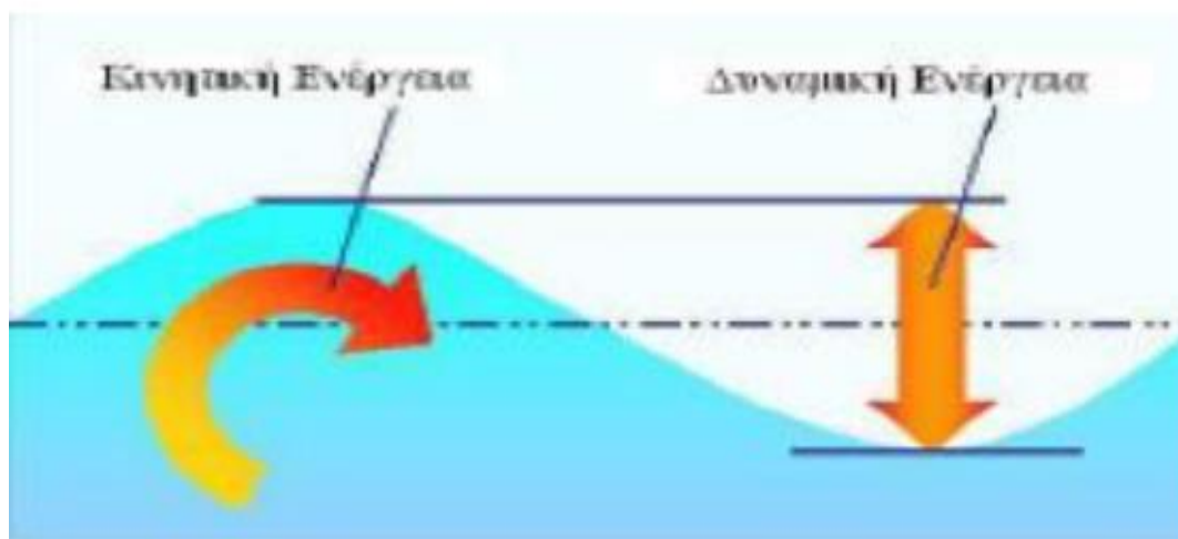
Εικόνα 1.5: Κατεύθυνση κινητικής και δυναμικής ενέργειας κύματος.
