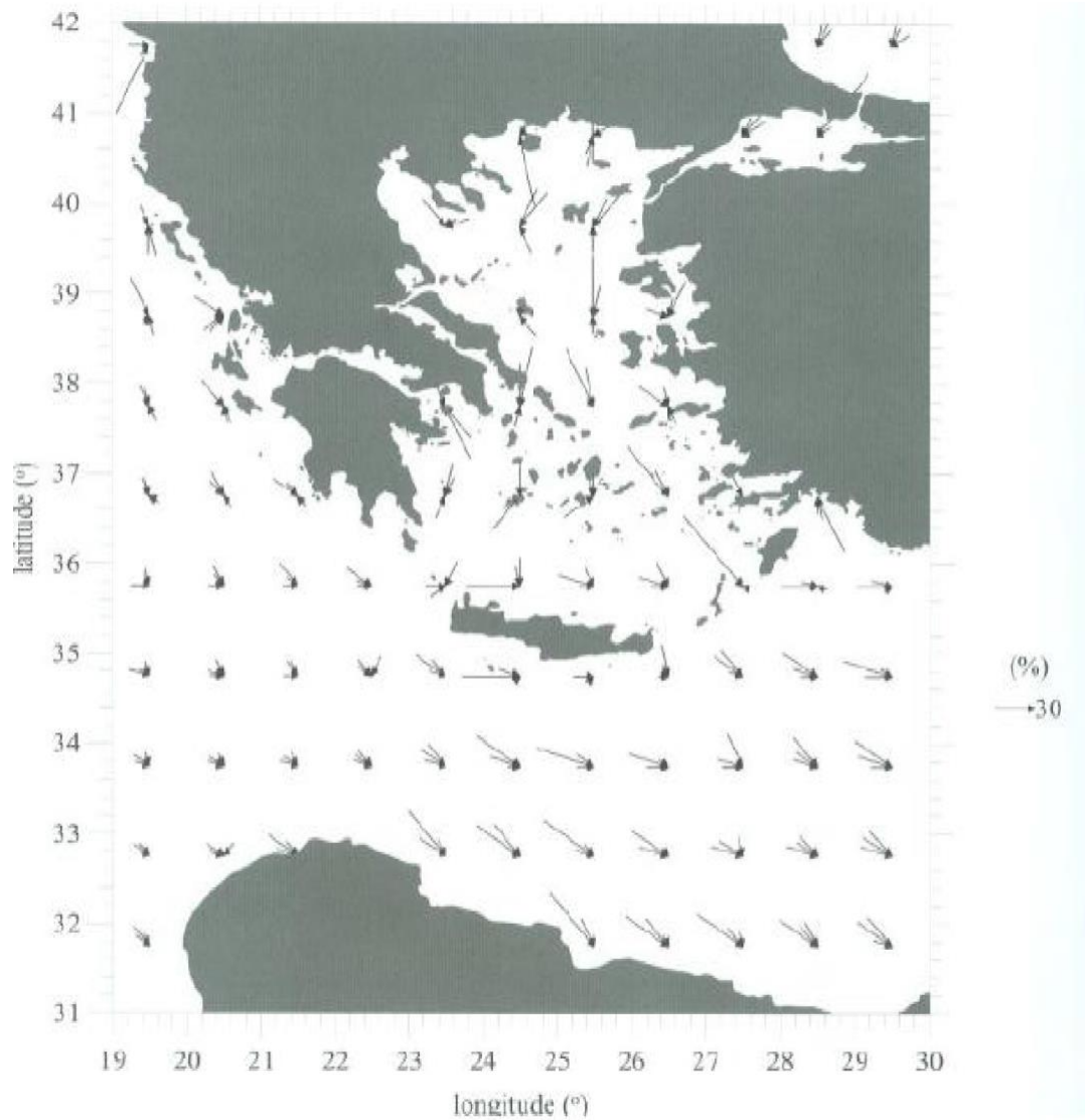
Εικόνα 5.6: Χωρική κατανομή της κατεύθυνσης των κυμάτων.
