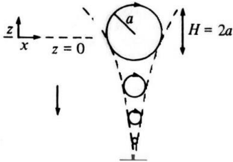
Εικόνα 1.3: Εδώ φαίνεται η κυκλική κίνηση στοιχειώδους μάζας νερού με ακτίνα κίνησης που ελαττώνεται σχεδόν εκθετικά όσο αυξάνεται το βάθος του.
