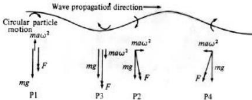
Εικόνα 1.4: Δυνάμεις σε επιφανειακά σώματα νερού στην επιφάνεια της θάλασσας.
