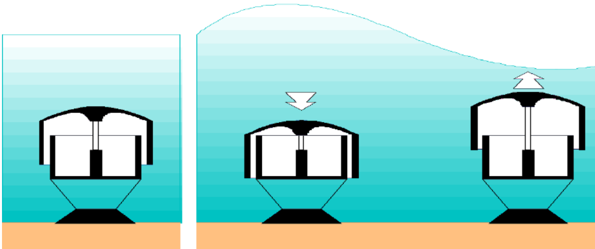
Εικόνα 4.21: Η βασική αρχή λειτουργίας του μετατροπέα AWS με την έλευση των θαλάσσιων κυμάτων.
