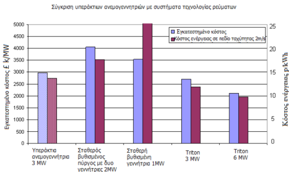
Εικόνα 3.8: Σύγκριση τεχνολογιών παραγωγής ηλεκτρικής ενέργειας.
