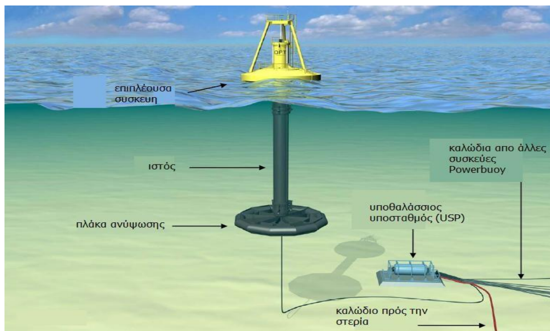
Εικόνα 4.24: Ο MKE Powerbuoy με τα επιμέρους συστήματα σύνδεσης με την στεριά.
