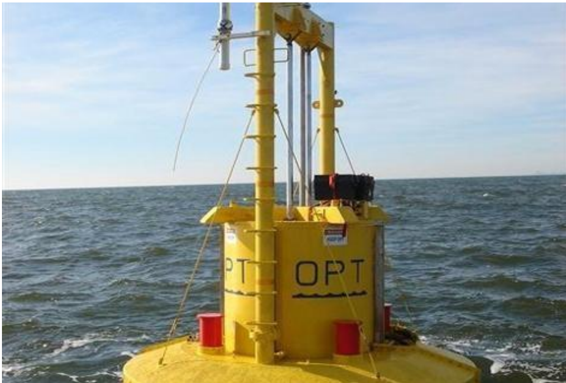
Εικόνα 4.23: Μοντέλο PowerBuoy των 40kW σε τοποθεσία δοκιμής στην ανοιχτή θάλασσα.
