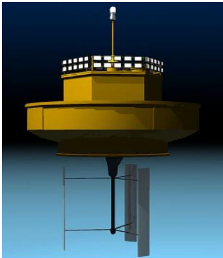
Εικόνα 3.11: Η τουρμπίνα κάθετου άξονα Kobold.
