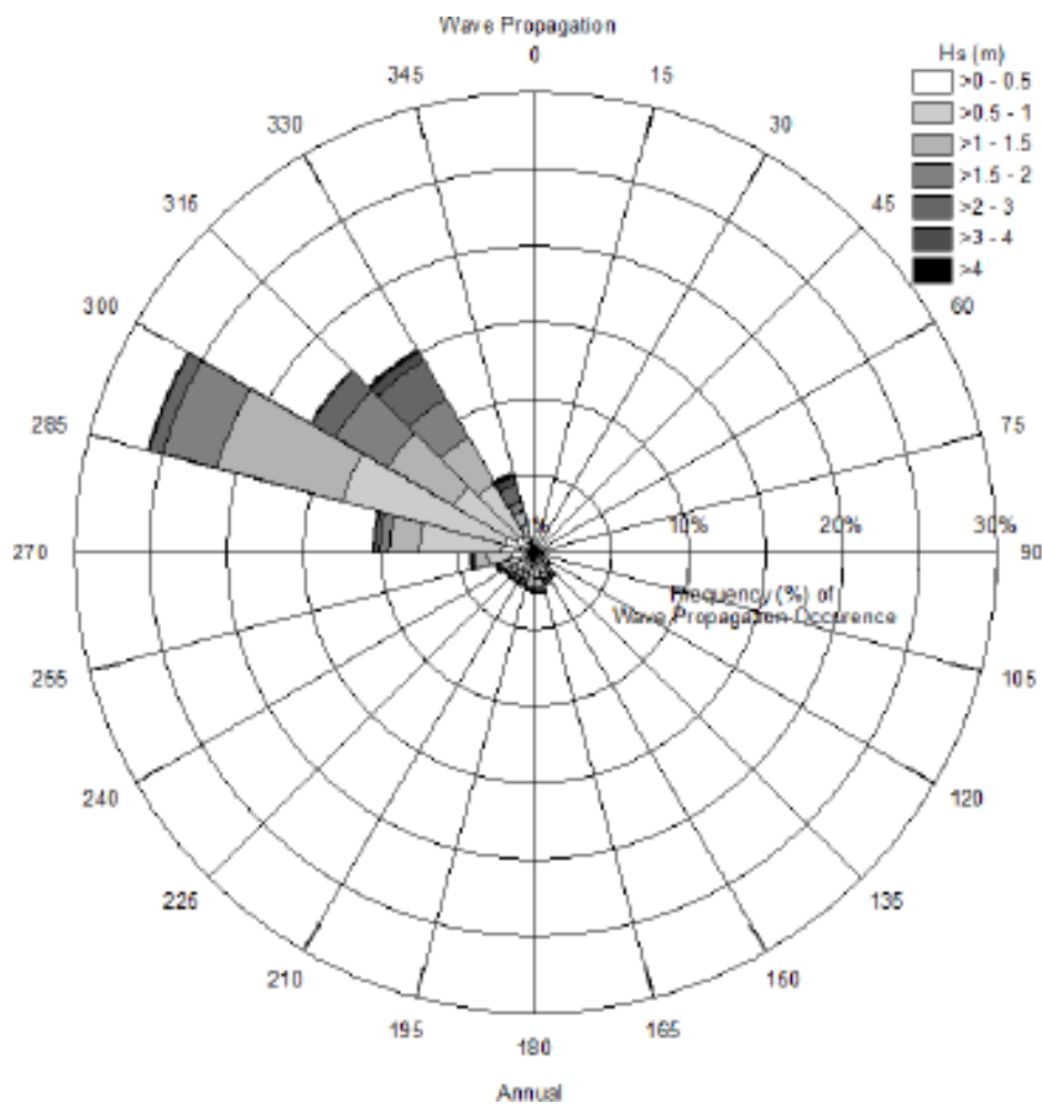
Εικόνα 5.3: Ετήσιο κυματικό διάγραμμα για την περιοχή μεταξύ Κάσου – Κάρπαθου.
