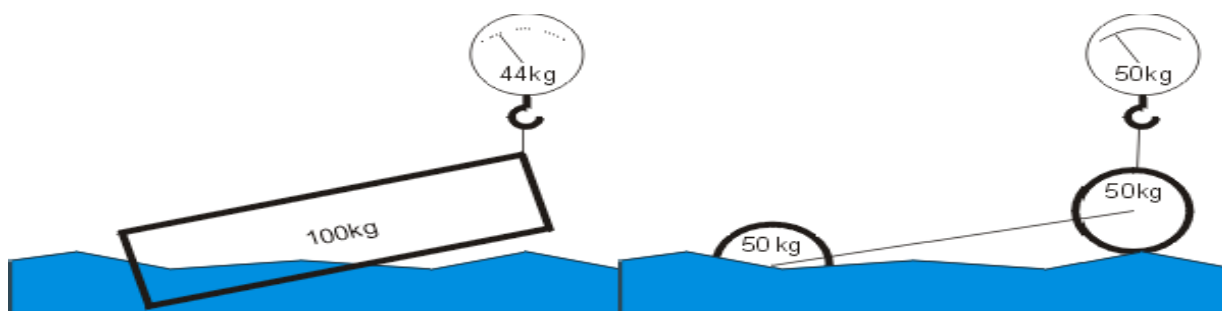
Εικόνα 4.32: Το πλεονέκτημα της κατανομής του βάρους του DEXA ως προς το Cockerell Raft.
