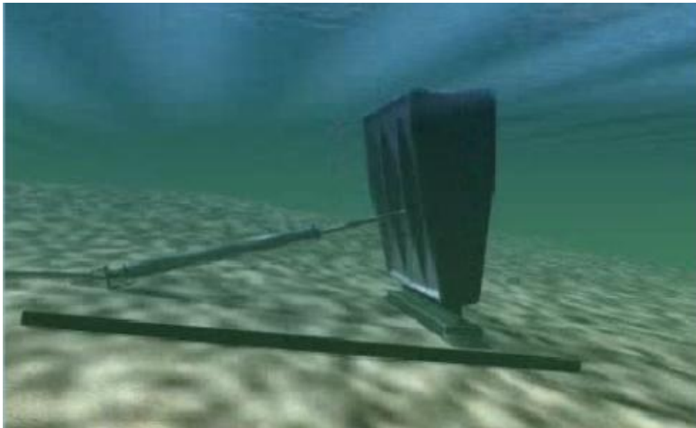
Εικόνα 4.38: Μια μονάδα μετατροπής WaveRoller. Διακρίνονται τα τρία βασικά της τμήματα, δηλαδή το περύγιο, η αντλία και η βάση εγκατάστασης.
