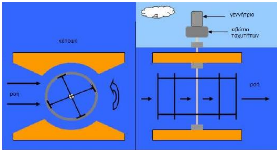
Εικόνα 3.9: Τουρμπίνα κάθετου άξονα με περίβλημα.
