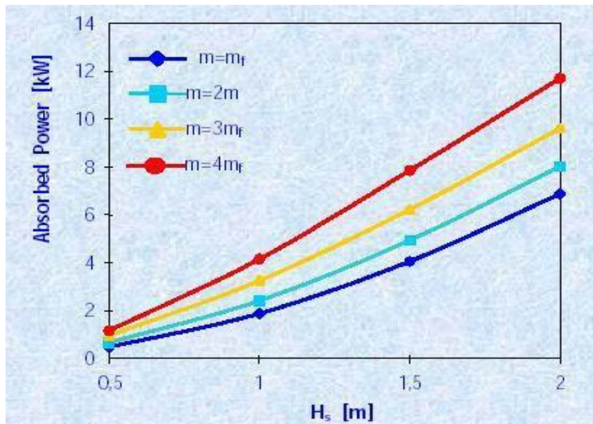
Εικόνα 4.15: Σχεδιάγραμμα της εξάρτησης της αποδοτικότητας σύλληψης της κυματικής ενέργειας από την αδράνεια του πλωτού σώματος του μετατροπέα (διάμετρος πλωτού σώματος 1,5 μετρα, βύθισμα ενός μέτρου, m_f=1,8 t).
