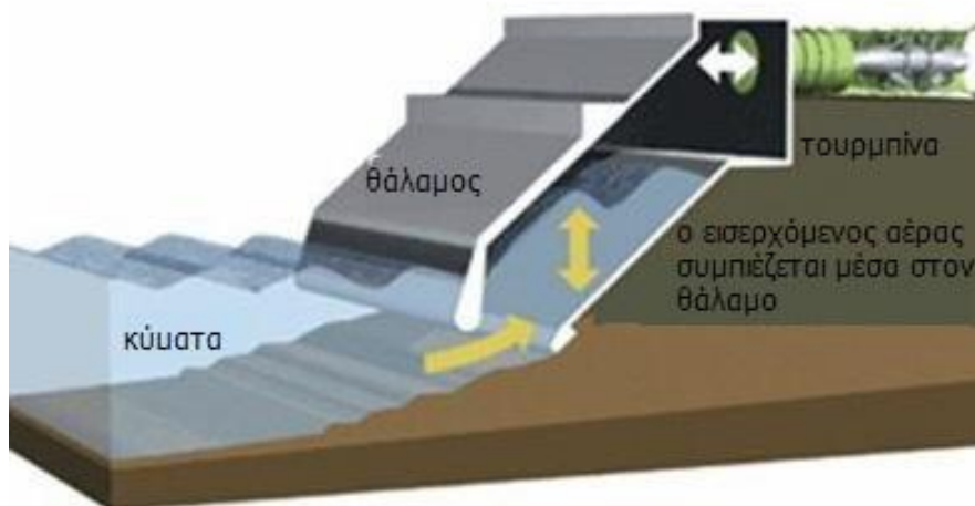
Εικόνα 4.1: Παράδειγμα διάταξης ταλαντευόμενης στήλης ύδατος.
